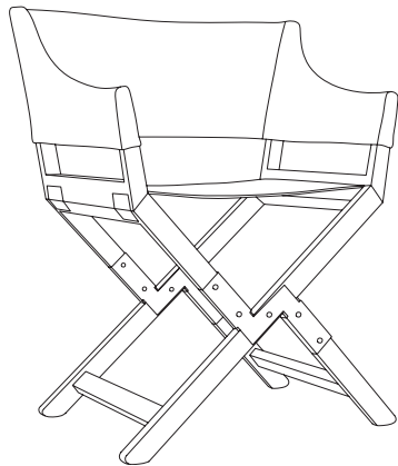
Schema di Montaggio Housses -- Fabric Cover Assembly
