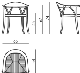
POLTRONCINA CON SEDILE INTRECCIATO ARMCHAIR WITH HANDWOVEN SEAT
