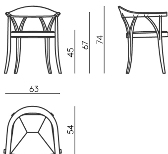
POLTRONCINA CON SEDILE IMBOTTITO ARMCHAIR WITH PADDED SEAT
